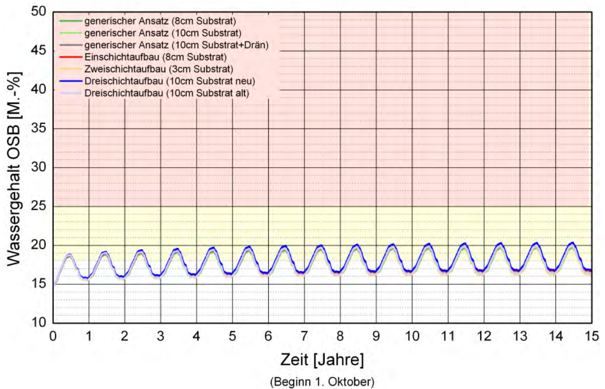
Bild 125: Berechneter Verlauf des Wassergehalts in der OSB-Platte einer Leichtbau- konstruktion mit 40 cm „Isofloc L“, raumseitiger OSB-Platte und 10 cm Überdämmung der äußeren Schalung in Abhängigkeit von verschiedenen Gründachaufbauten.
