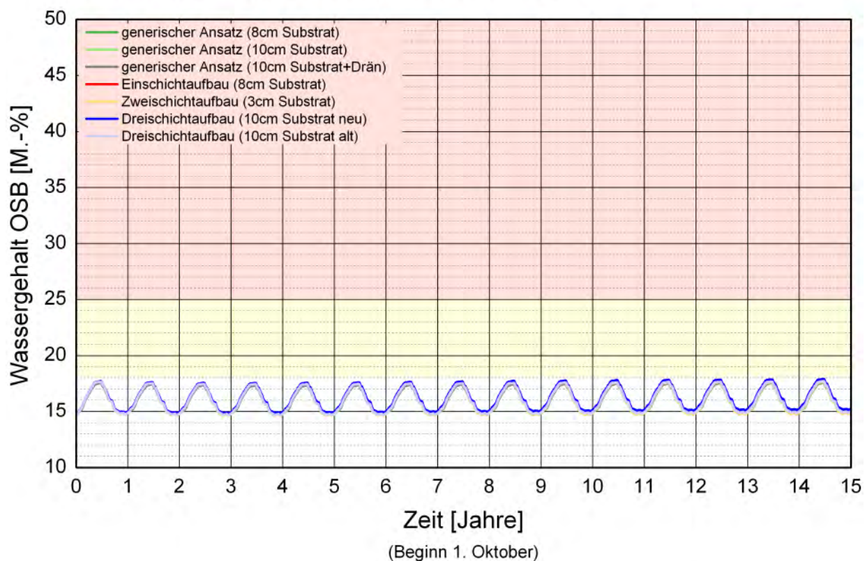
Bild 114: Berechneter Verlauf des Wassergehalts in der OSB-Platte einer Leichtbau- konstruktion mit 40 cm „Isofloc L“, raumseitiger „INTELLO“ und 15 cm Überdämmung der äußeren Schalung in Abhängigkeit von verschiedenen Gründachaufbauten.
