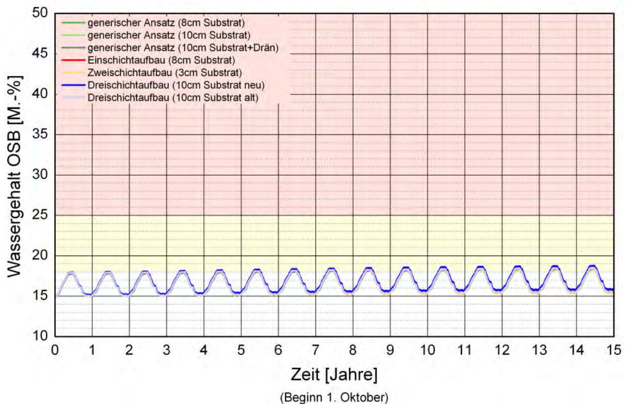
Bild 113: Berechneter Verlauf des Wassergehalts in der OSB-Platte einer Leichtbau- konstruktion mit 40 cm „Isofloc L“, raumseitiger „INTELLO“ und 12 cm Überdämmung der äußeren Schalung in Abhängigkeit von verschiedenen Gründachaufbauten.
