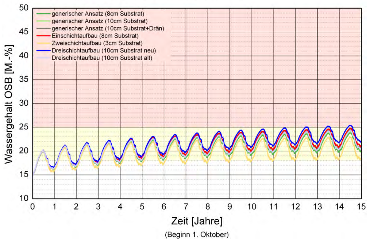
Bild 110: Berechneter Verlauf des Wassergehalts in der OSB-Platte einer Leichtbau- konstruktion mit 40 cm „Isofloc L“ und raumseitiger „INTELLO“ ohne Überdämmung der äußeren Schalung in Abhängigkeit von verschiedenen Gründachaufbauten.
