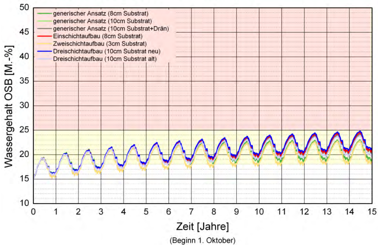
Bild 115: Berechneter Verlauf des Wassergehalts in der OSB-Platte einer Leichtbau- konstruktion mit 20 cm „Isofloc L“ und raumseitiger „Vario Xtra“ ohne Überdämmung der äußeren Schalung in Abhängigkeit von verschiedenen Gründachaufbauten.
