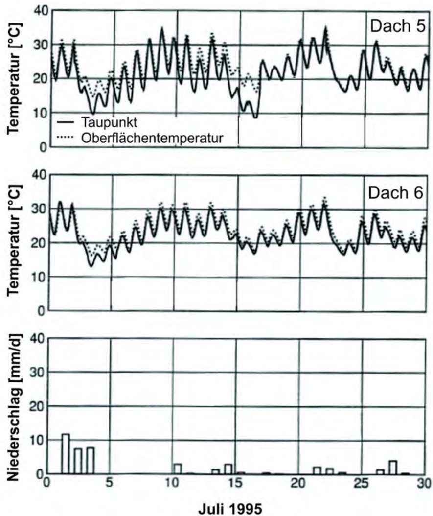
Bild 3: Gemessener Verlauf von Temperatur (gestrichelte Linie) und Taupunkttemperatur (durchgezogene Linie) unter der Kiesschicht von Dach 5 (oben), unter der Blähtonschicht von Dach 6 (mitte) sowie die gemessene Niederschlagsmenge für Juli 1995.
