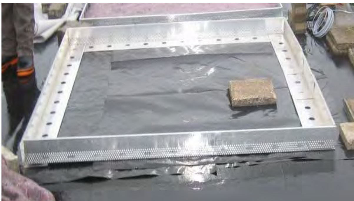
Dachaufbau 3:
